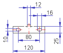
Ansicht "Y"
